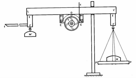
Schéma du dispositif d'essais de G.A.Hirn (1854)
